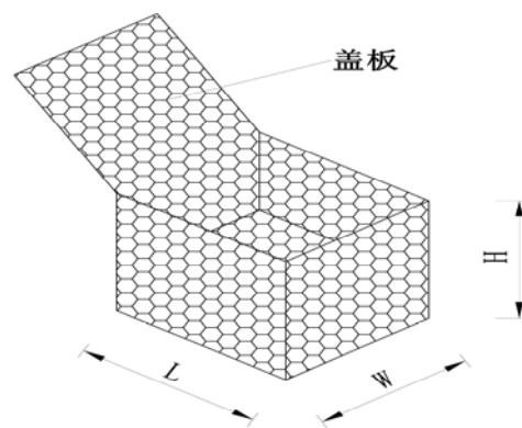
图8 网箱
