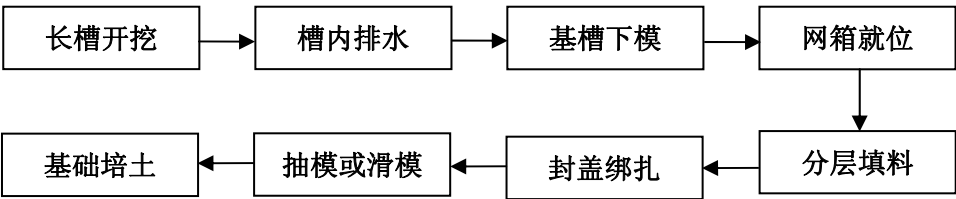
图15 格宾网箱基础干法施工工序流程图
