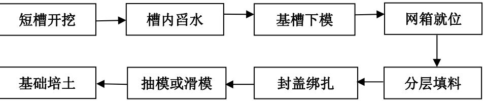
图16 格宾网箱基础水下施工工序流程图
