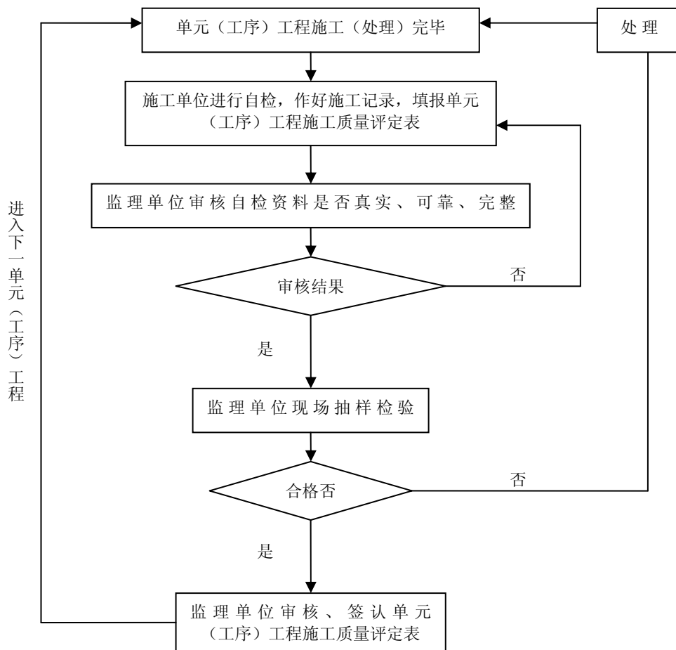
单元工程质量检验工作程序图
