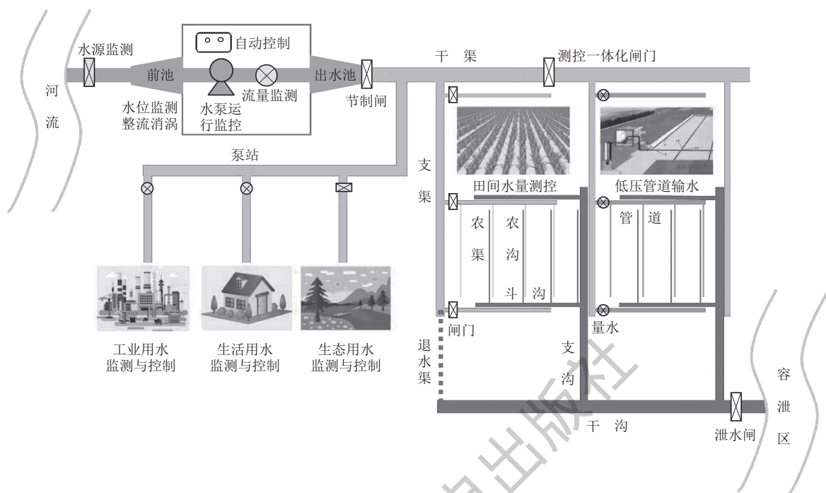
图 A 提水灌区用水全程量测控概化图
